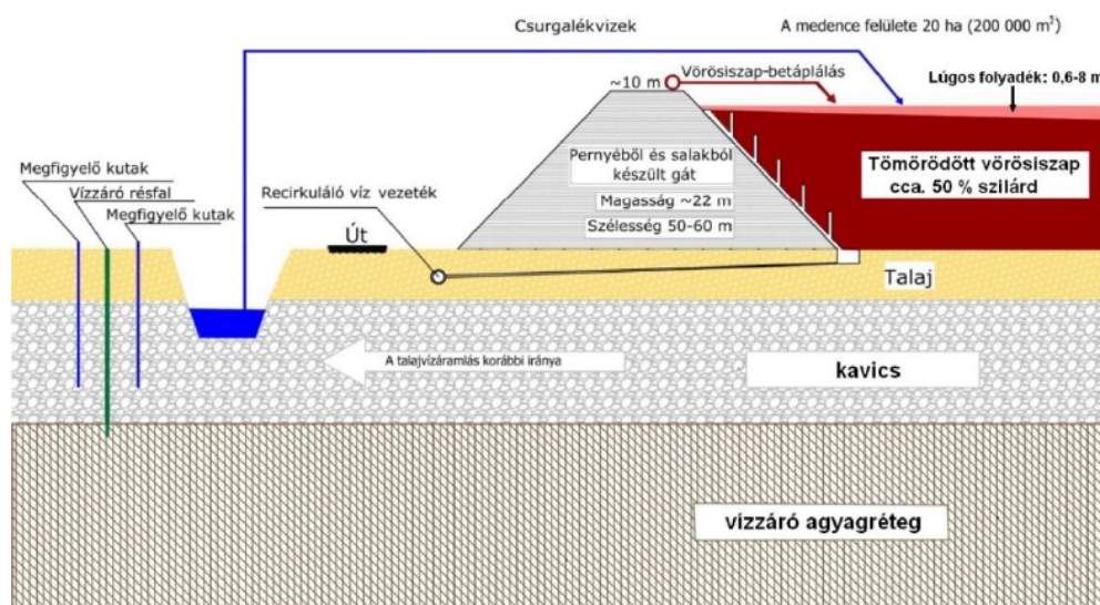
1. ábra. A gát és a kapcsolódó létesítmények elvi keresztmetszésvénye [A schematic of the red mud disposal system] (Baksa Gy. & Kajdi S., 1992, módosította Bánvölgyi Gy., 2010)
